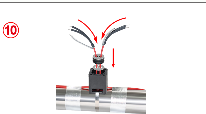
10 : Remplir l'entrée des manchons isolant de silicone liquide. Glisser les manchons isolants sur les conducteurs des cables chauffants, en laissant le conducteur de terre en dehors. Puis glisser ensuite le tube de protection sur les conducteurs de terre.
