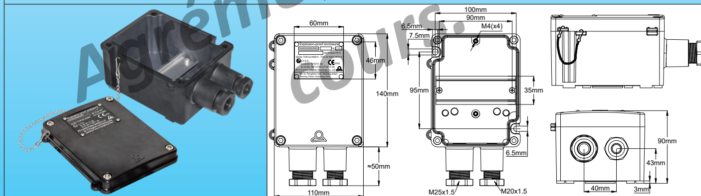
Exemple avec seulement rail DIN
